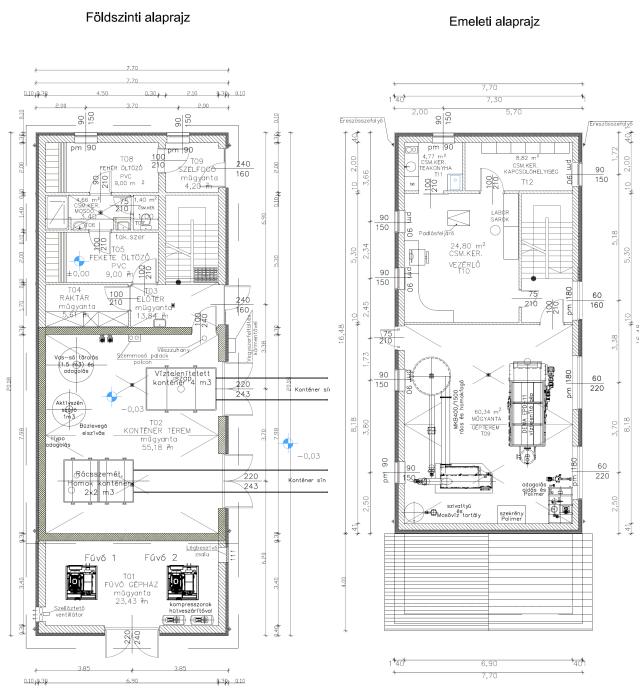
Technológiai épület földszinti és emeleti alaprajzai
